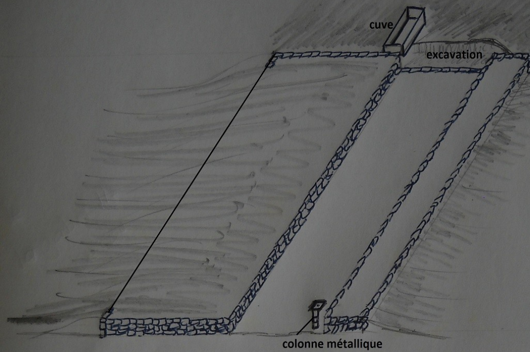
perspective de la sécherie
